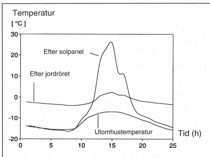
Figur 2. Temperaturer ute, före och efter jordröret, studie 2, (5).
