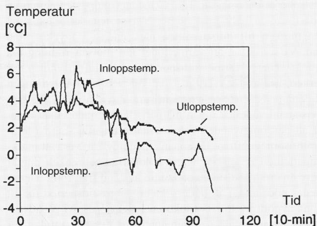
Figur 1. In- och utloppstemperaturer för jordröret första veckan i januari 1988.
