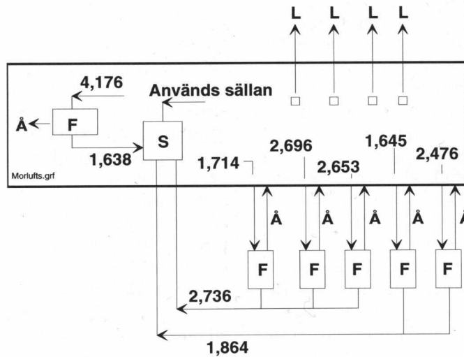
Figur 5. Spånsugsystem.
