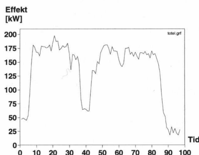
Figur 3. Ånganläggning.
