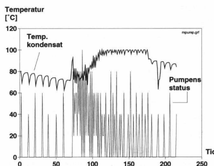
Figur 4. Kondensatets temperatur samt pumpens status 1998-04-16 kl 00.00 till 17.55.
