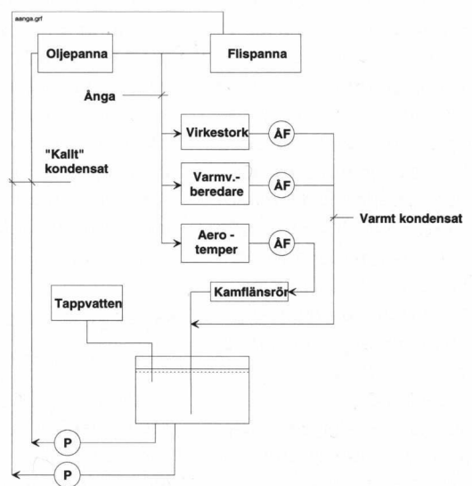
Figur 3. Ånganläggning.
