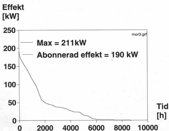
Figur 1. Varaktighetsdiagram för elanvändning 1997.
